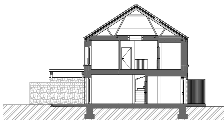
ŘEZ
